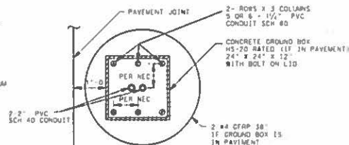
DETAIL A4
